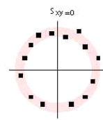
Hay dependencia entre las dos variables, aunque la covarianza sea nula.
