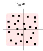
Las dos variables son independientes.
